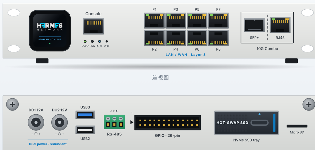
後視圖
